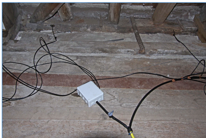
Drukloos injecteren van muurplaten met aantasting door de bonte knaagkever (grote houtwormkever)
