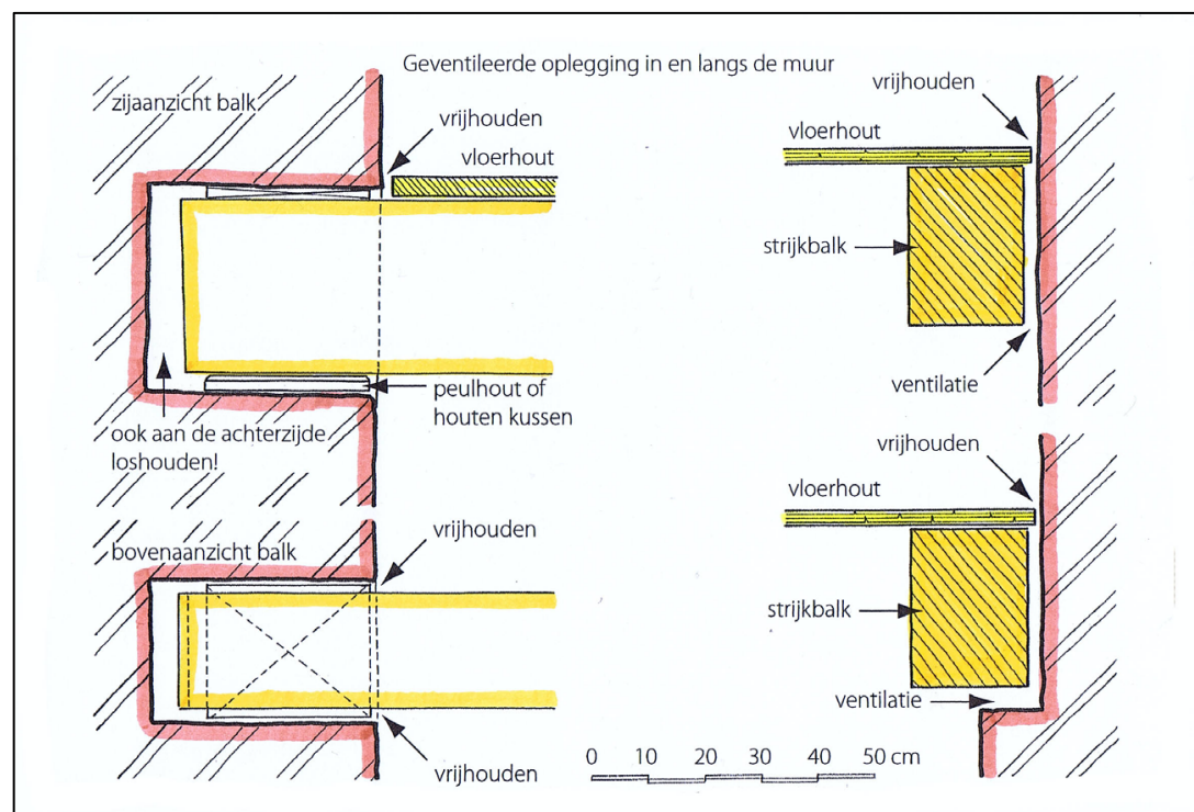
Figuur 3 Geventileerde oplegging van balkkoppen en strijkbalken
