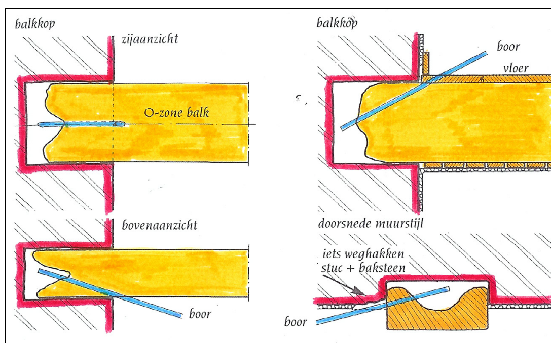
Figuur 1 Inspectiemethode bij boren in balkkoppen en muurstijlen
